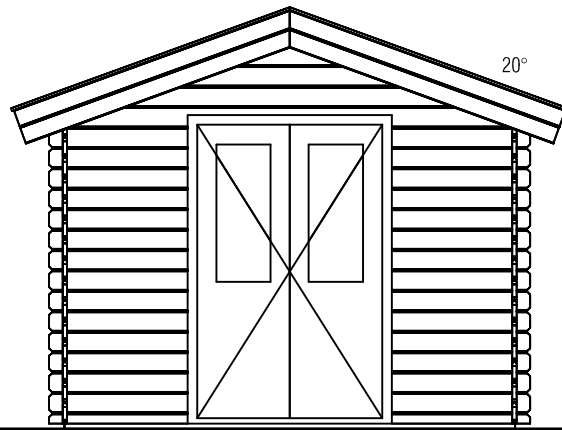
Vooraanzicht / Front view / Vorderansicht
