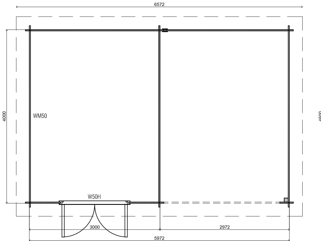
Plattegrond / Plan
