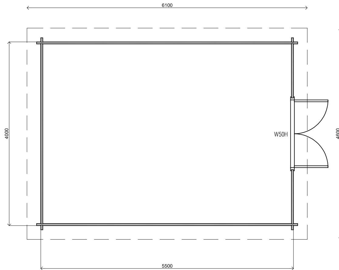
Plattegrond / Plan
