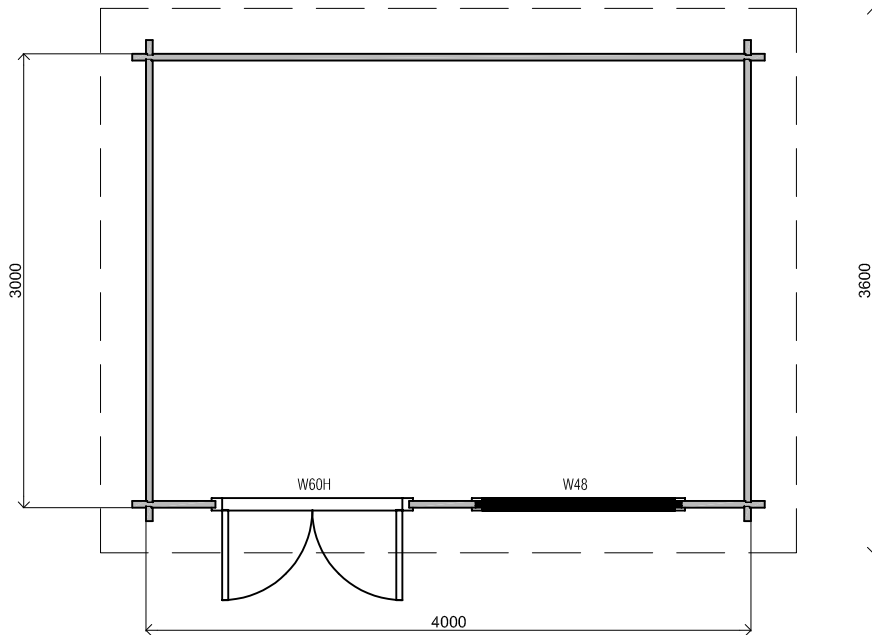
Plattegrond / Plan
